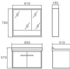
ACBA-T036-80B Main Cabinet : 850 × 510 × 570 mm Mirror Cabinet : 810 × 180 × 780 mm
