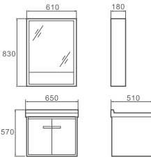
ACBA-T036-60B Main Cabinet: 650× 510 × 570 mm Mirror Cabinet : 610× 180× 830 mm
